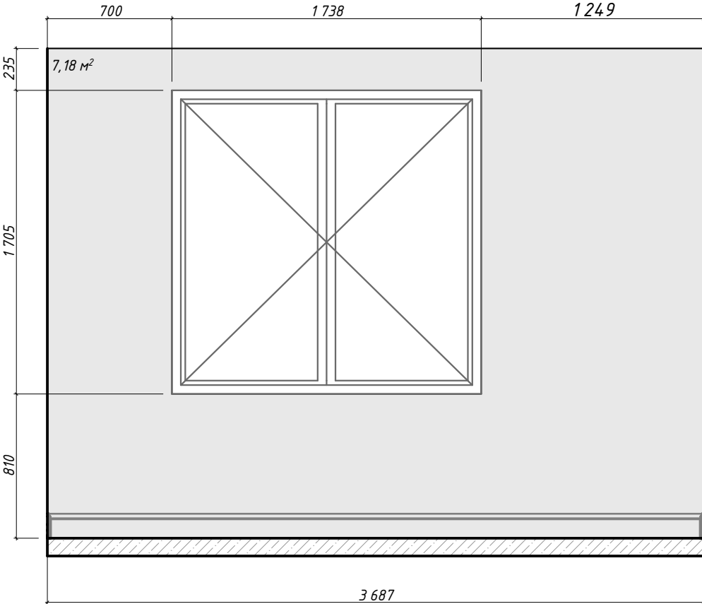
Стена 07
