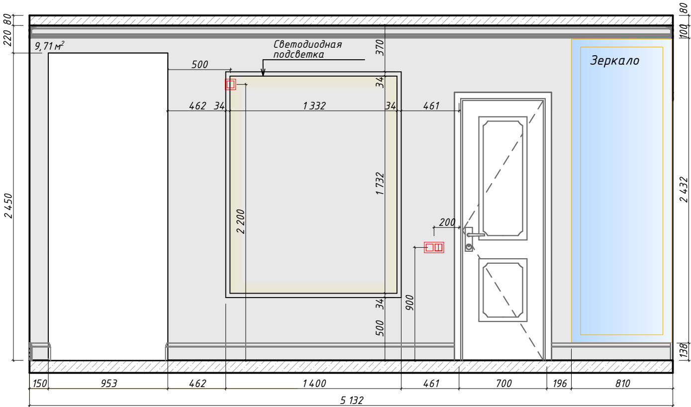
Стена 04
