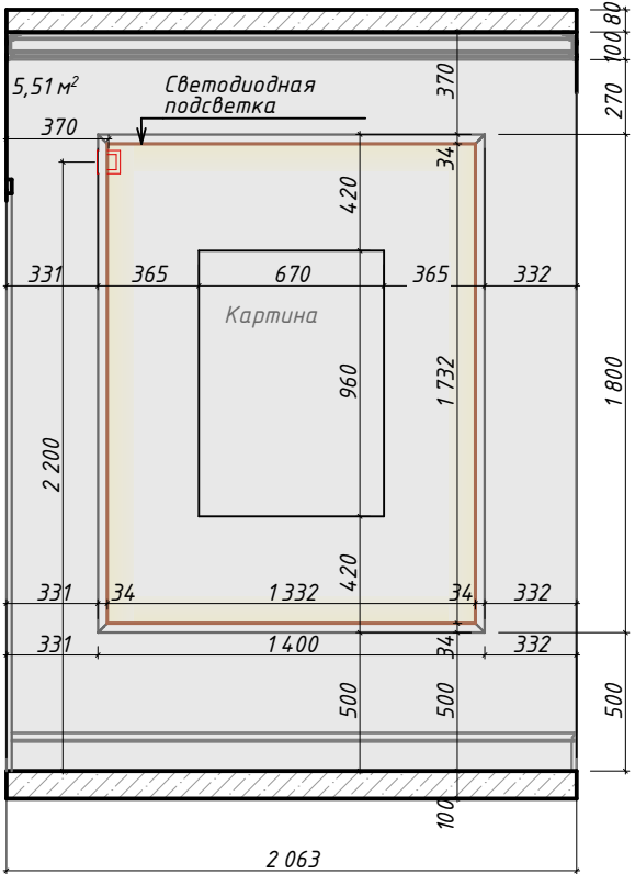
Стена 03
