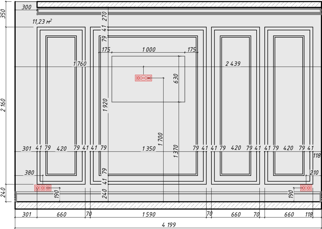
Стена 04
