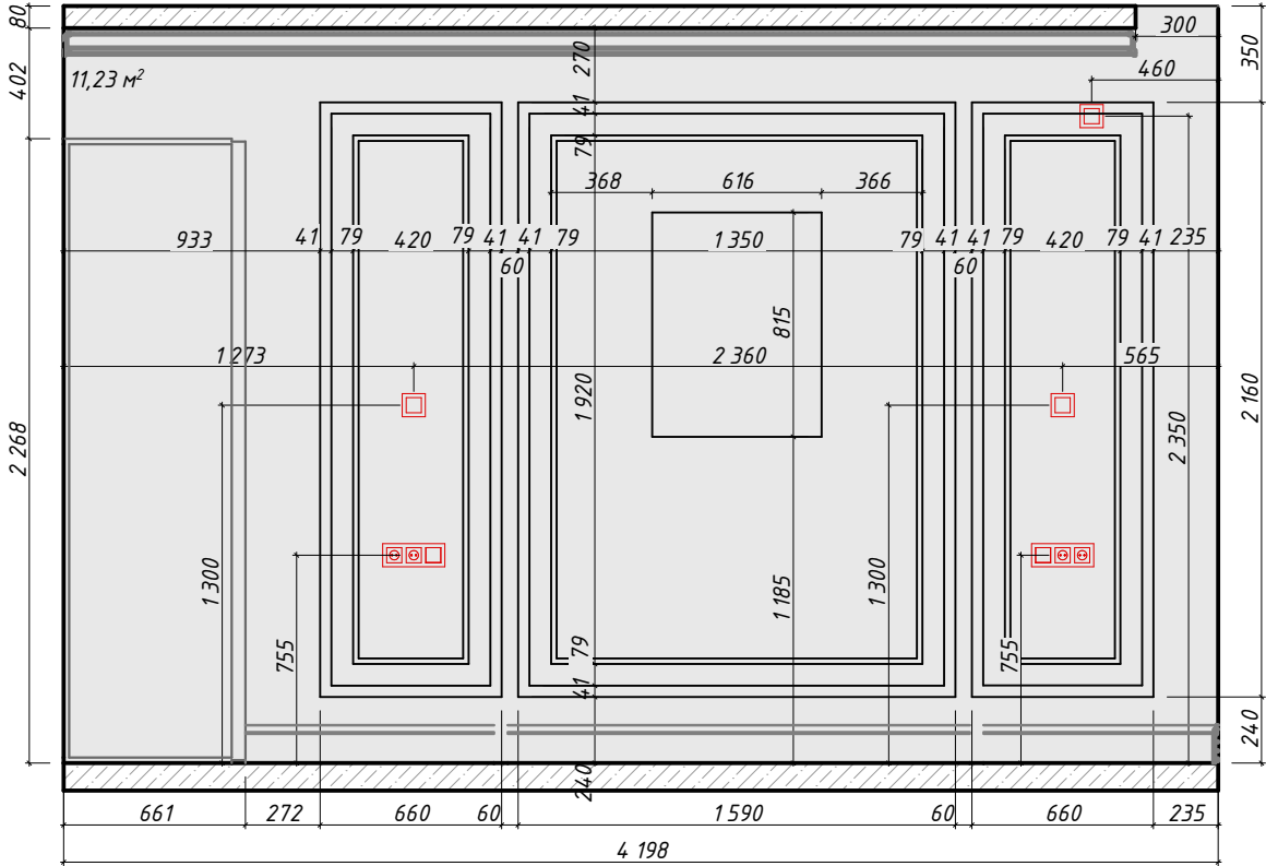
Стена 04
