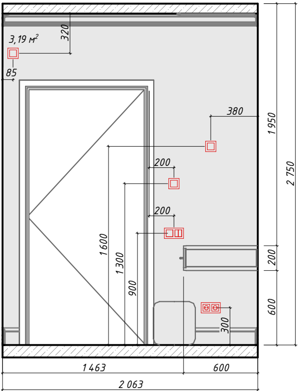
Стена 01
