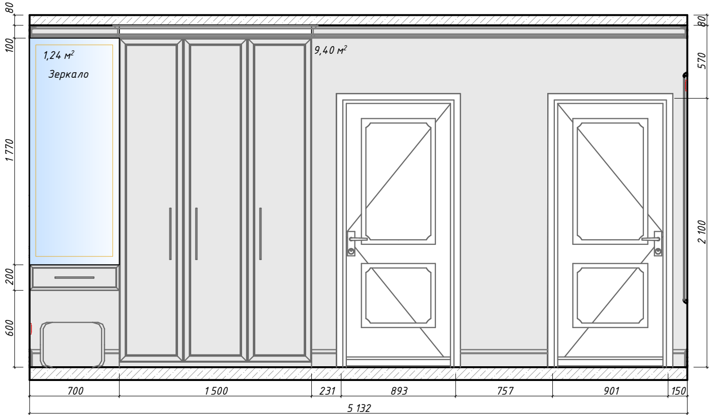
Стена 02
