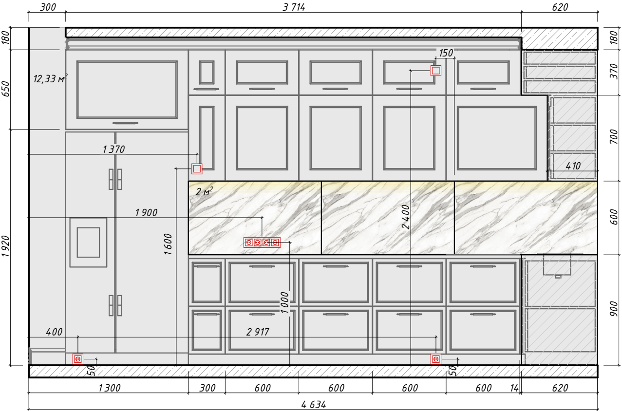
Стена 08
