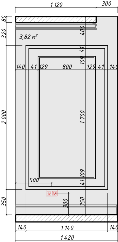
Стена 09
